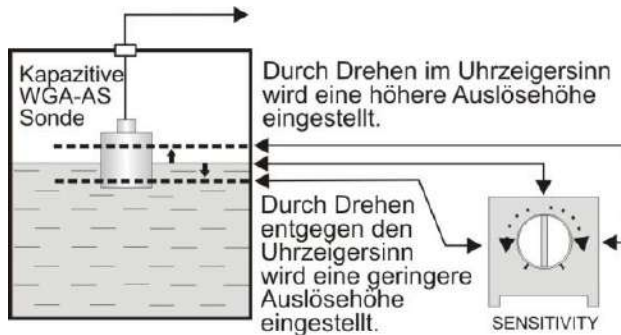
Abbildung 9. Auslösehöhe einstellen
