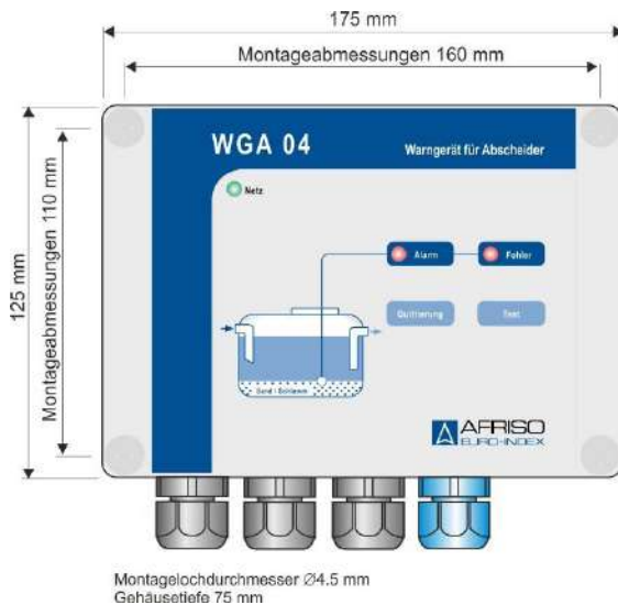
Abbildung 2. Abmessungen, WGA 04 Steuereinheit
