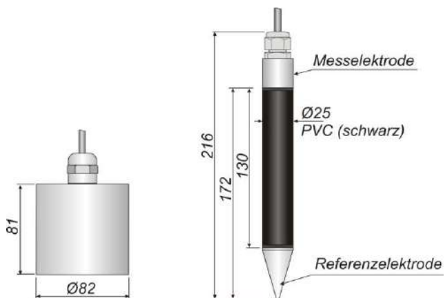
Abbildung 3. Maßblatt für WGA-AS (links) und WGA-SD 03 (rechts)
