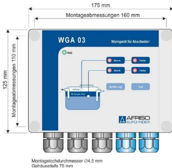
Abbildung 2. Abmessungen, WGA 03 Steuereinheit
