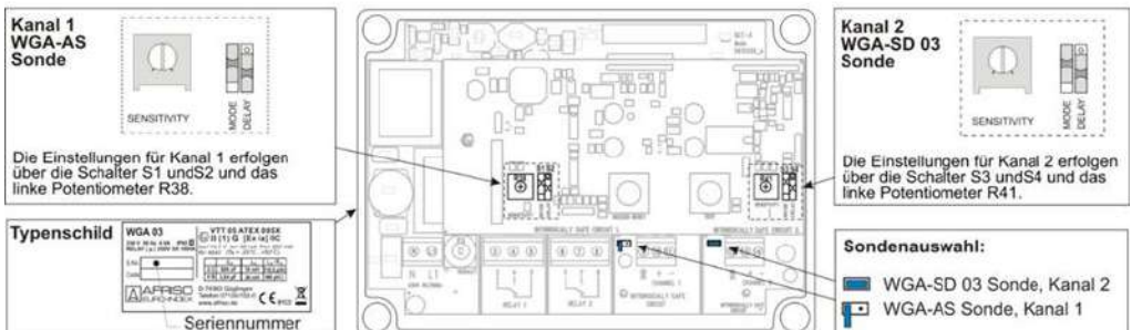
Abbildung 6. Werkseinstellungen des WGA 03
