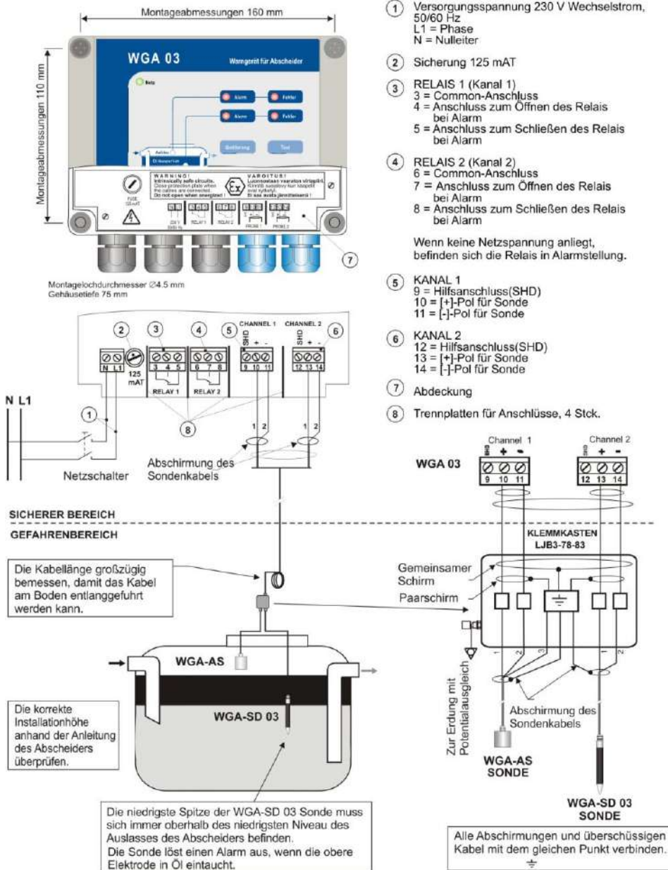
Abbildung 5. Installation des WGA 03 Warngeräts
