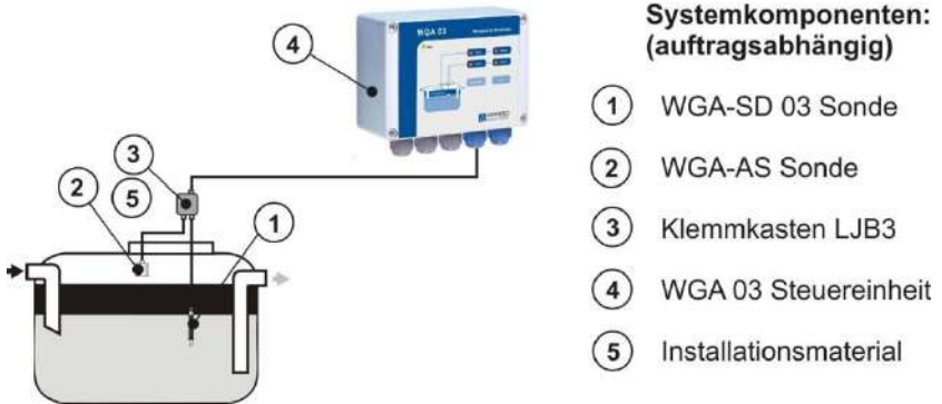
Abbildung 4: Alarmsystem für Ölabscheider mit WGA 03
