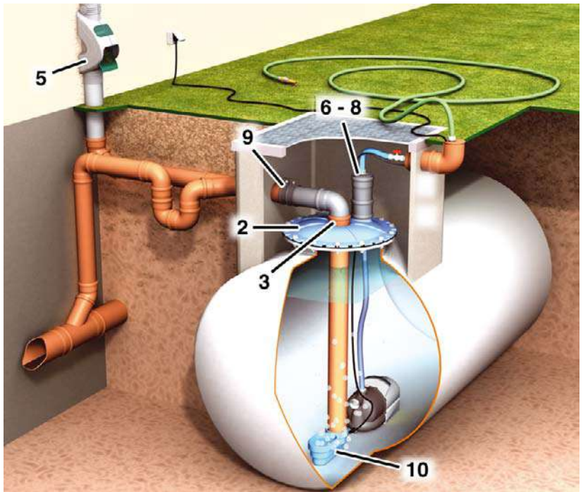
Bild 2: Öltank-Umrüstset II
