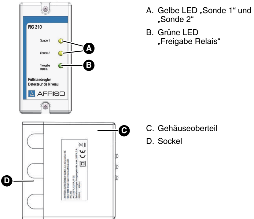
Abbildung 1: Füllstandregler
