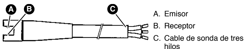
Figura 1: Sonda opto-electrónica
