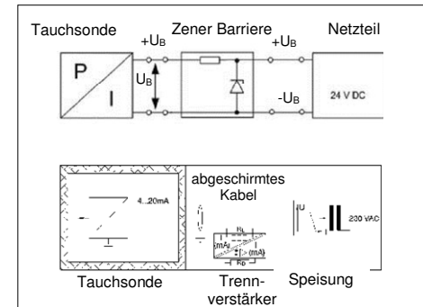
Abb. 5 Schaubilder Beschaltung
