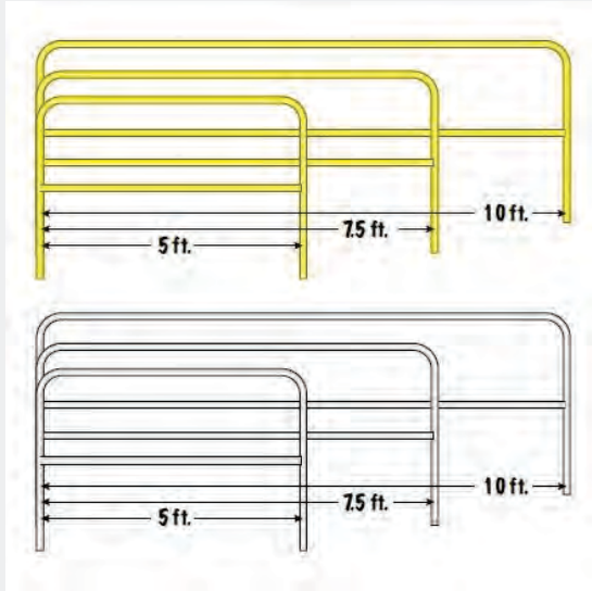
Roof Edge Railing
