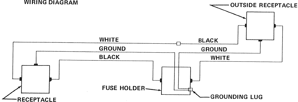
110 VOLT WIRING DIAGRAM
