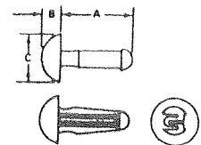
203-925 Accordion rivet.
