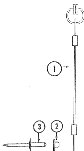
SCREEN DOOR CABLE ASS'Y 4734B5211
