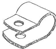
TUBE CLAMPS 1201-870 3/8" St./Neo. 1201-873 1/2" St./Pl. 4739-425 3/8" Alum.
