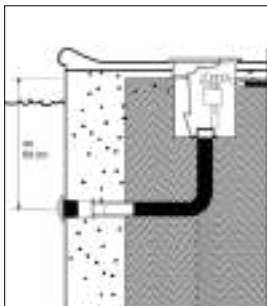
Esquema Regulador de Nível
