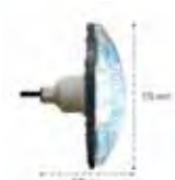
Projetor a roscar num passamuro de parede de 1.5''
