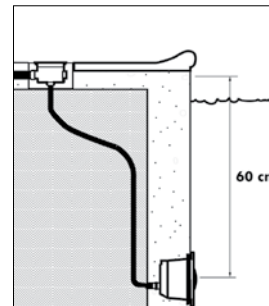
Esquema Projetor
