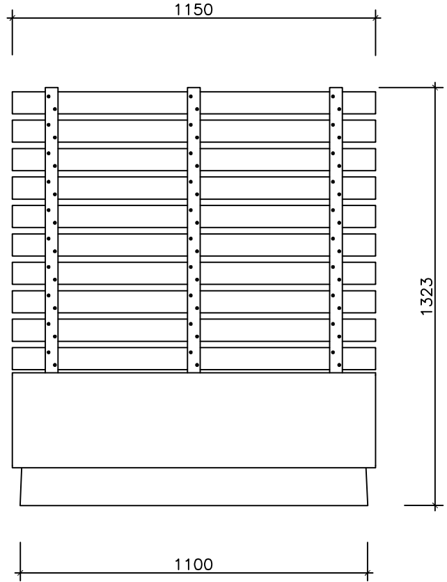
ALÇADO Side View
