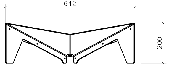
ALÇADO Side View
