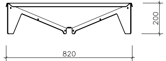
ALÇADO Side View
