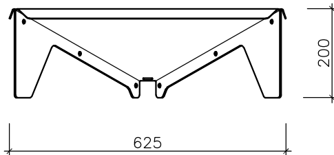
ALÇADO Side View
