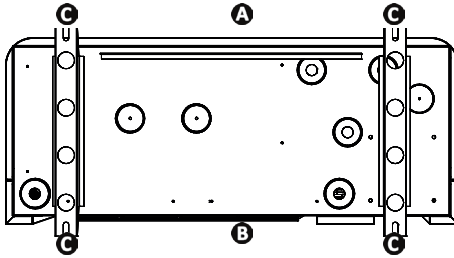
Onderaanzicht van het voetstuk van het apparaat voor het installeren van de trillingsdempers
