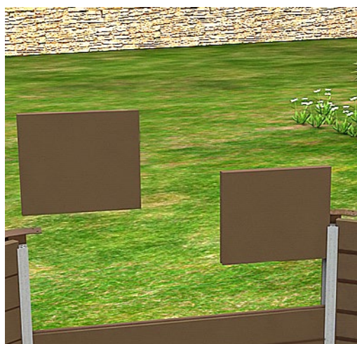
Colocação da travessa nº 5
