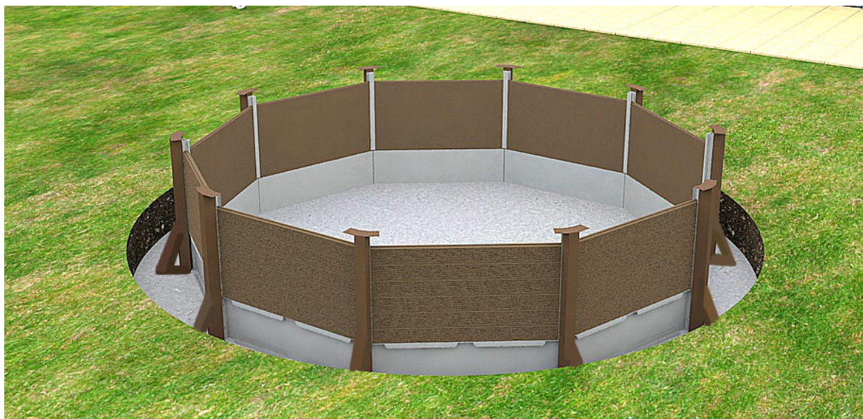
Colocação da travessa nº 2 até à fiada nº 6.
