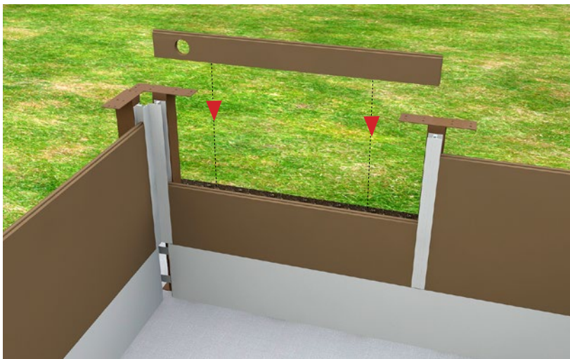
Traviesa nº 4
