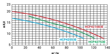
CURVAS DE RENDIMENTO / BOMBA HCP4200
