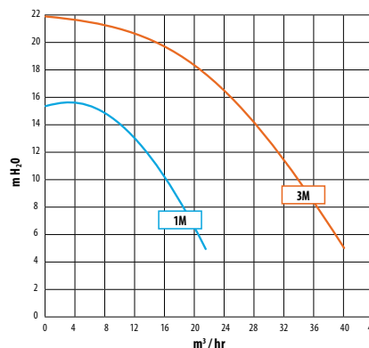
CURVAS DE RENDIMENTO / BOMBA SILEN PLUS
