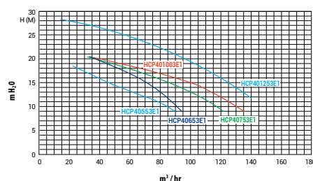
CURVAS DE RENDIMENTO / BOMBA HCP4000
