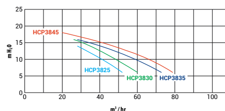
CURVAS DE RENDIMENTO / BOMBA HCP3800
