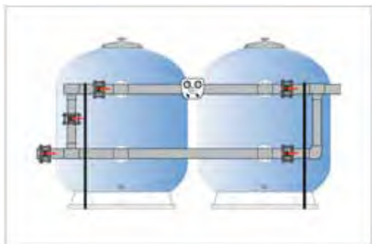
Esquema de instalação dupla
