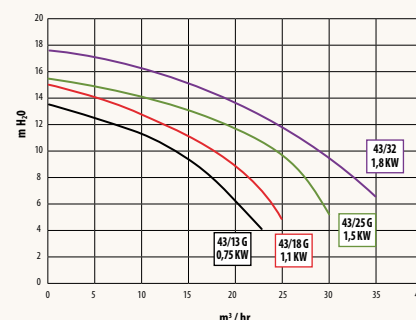
CURVAS DE RENDIMENTO / BOMBA STA-RITE 5P6R
