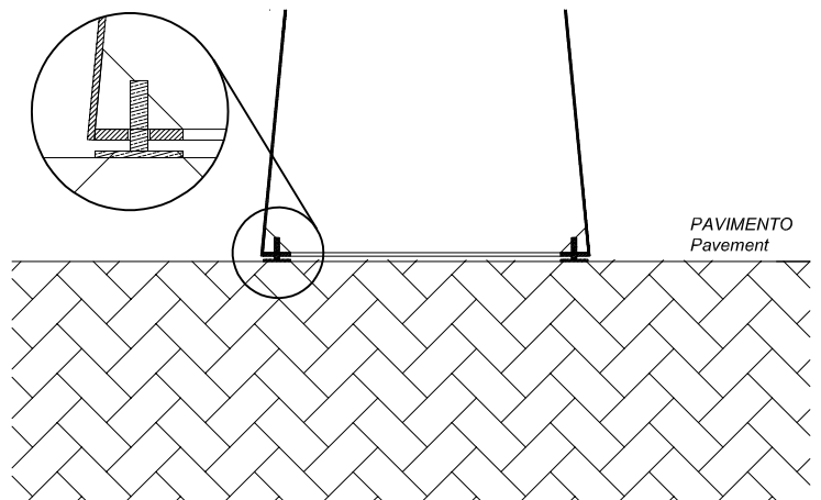
2 - SIMPLEMENTE APOIADO NO SOLO COM NIVELADOR Self Standing with leveler
