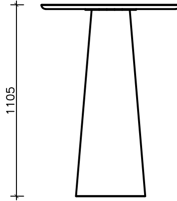
ALÇADO Side View
