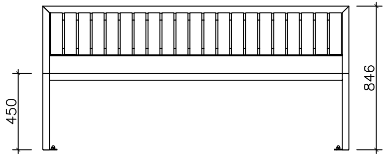
ALÇADO FRONTAL Front View
