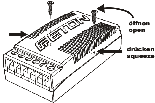
Abbildung 5 Figure 5 Montage der Weiche Installing the crossover
