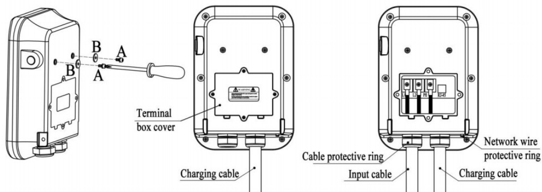
Fig. 5-3 Wiring
