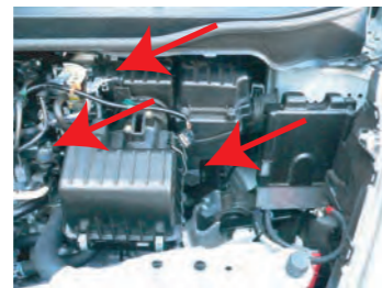
5. スロット部分のバンドと2箇所ボルトを外しクリーナーケースを取り外します。
