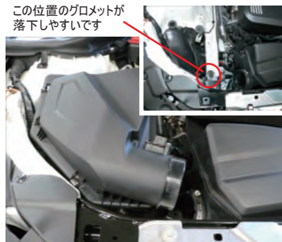
エアークリナーボックスを取り出します。(グロメットの落下に注意してください)
