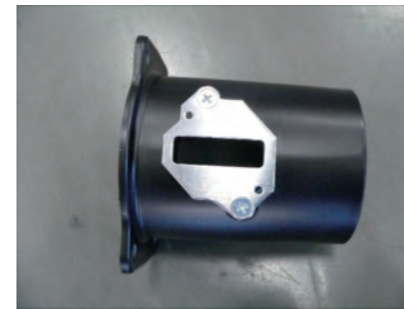
センサーアダプターに変換プレートを皿ビス2本で固定します。
