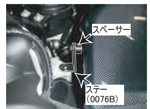
17: 右側のダクトを固定します。ステーとダクトの間にスペーサーを挟みビスCで固定。ボディ側はビスBで固定。
