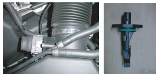
3: エアフロセンサーを付属レンチでネジを緩めて、取り外します。
