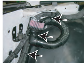
6: ウォッシャータンクノズルをタイラップで固定します。
