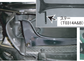
13: 導入ダクトをバンパー裏にステーT0314AとT0314Bで取り付けます。
