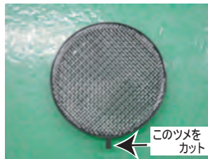
8: 取り出した整流ハニカムのツメをカットします。
