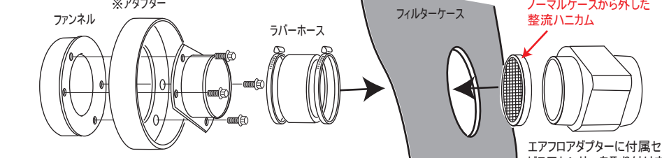
9: 付属パーツを図の通りに組み立てます。*アダプターの裏表の向きに注意。イラスト参照
