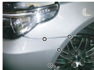
フェンダー&バンパー横部 (左右 各4ヶ所)
