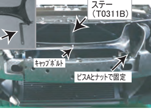
14: 導入ダクトのセンター部固定用のステー(T0311B)を取り付けます。ステー上側はバンパーと共締めします。下側はバンパーフレームと発泡スチロールの間に挟みます。
