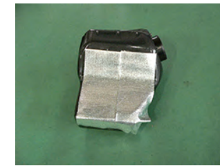
耐熱マットテープを貼り付いたら、ネジ部やカバーの合わせ部はカッターで切り込みを入れておきます。
