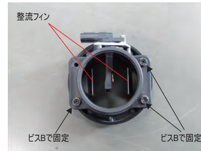
11. アダプターとセンサーアダプターの間に整流フィンを挟み、組付けます。
