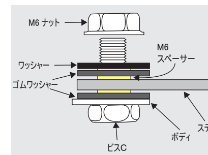
(ステア取付け部の詳細)
