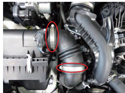
2. バンド2箇所緩め、サクシオンホースを取外します。(後で反転させて取り付けます)
