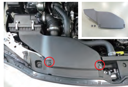
1. クリップを2箇所を外し、導入ダクトを取外します。
