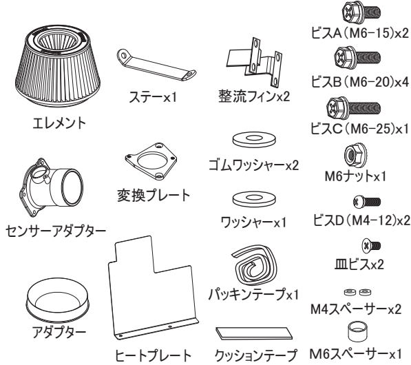
11. アダプターとセンサーアダプターの間に整流フィンを挟み、組付けます。
