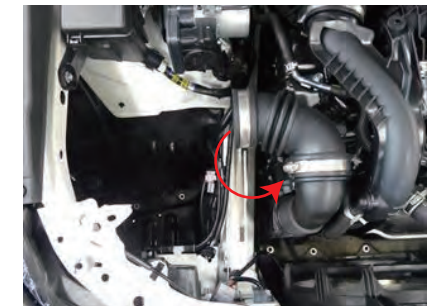
13. 純正サクシオンホースを反転させ、長さが短い方をパイプに取付けます。
