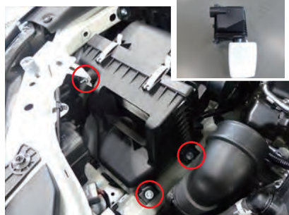
5. ボルト2箇所とナット1箇所を取外し、クリーナーボックスを取外します。
