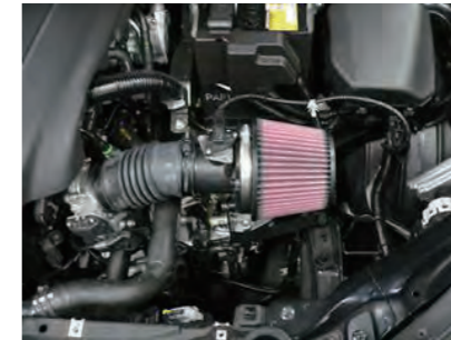
14. エレメントを取付けます。
