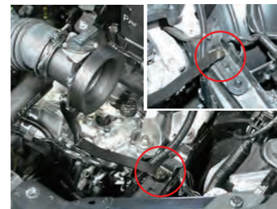
13. スペーサー 15mm を挟みステアをビス Cx1 で車両に固定します。
