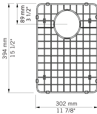
RGR800CAP - pour petit évier / for small sink Cabernet et Merlot 800D
