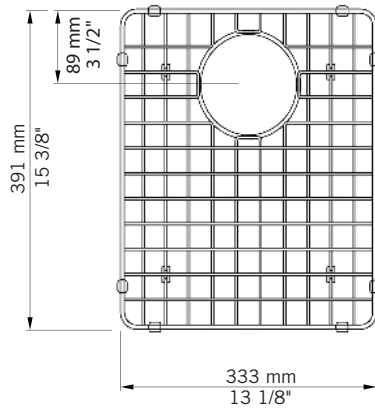
RGR370 - pour éviers / for sinks Cabernet & Merlot 370S
