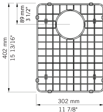
RGR800SYP - pour petit évier / for small sink Muscat et Syrah 800D
