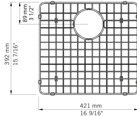
RGR800CAG - pour grand évier / for big sink Cabernet et Merlot 800D
