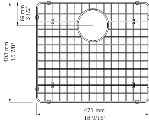
RGR540 - pour éviers / for sinks Muscat & Syrah 540S
