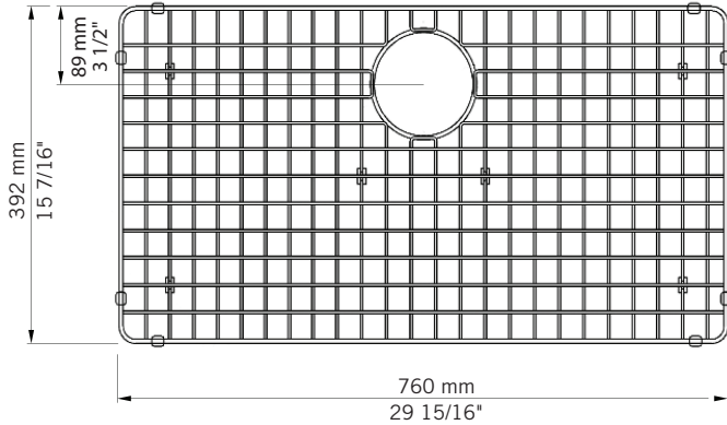
RGR800 - pour éviers / for sinks Cabernet et Merlot 800S
