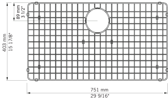
RGR820 - pour éviers / for sinks Muscat et Syrah 820S
