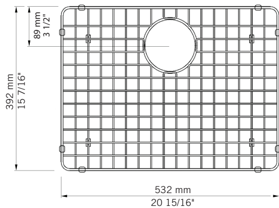
RGR570 - pour éviers / for sinks Cabernet & Merlot 570S
