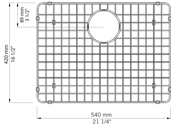
RGR575 - pour éviers / for sinks Gamay 575S
