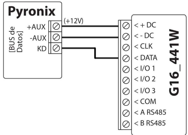
Diagrama de conexión de Pyronix con G16_441W
