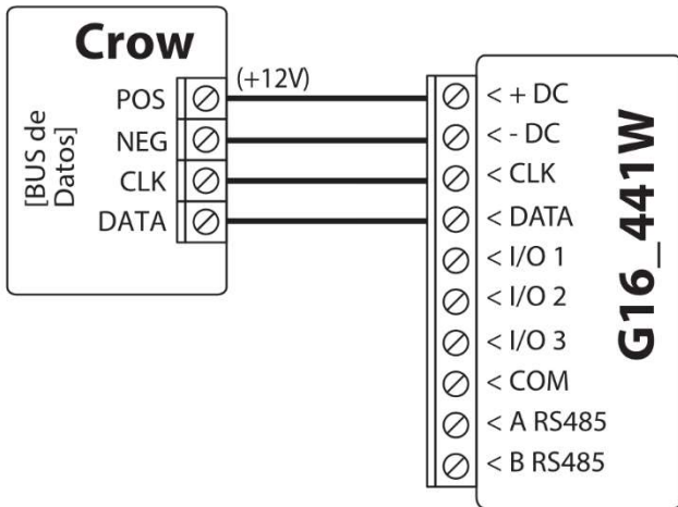
Diagrama de conexión de Crow Runner 4/8, Runner 8/16 con G16_441W
