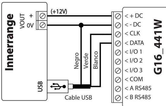
Diagrama de conexión de INNERRANGE INCEPTION con G16_441W
