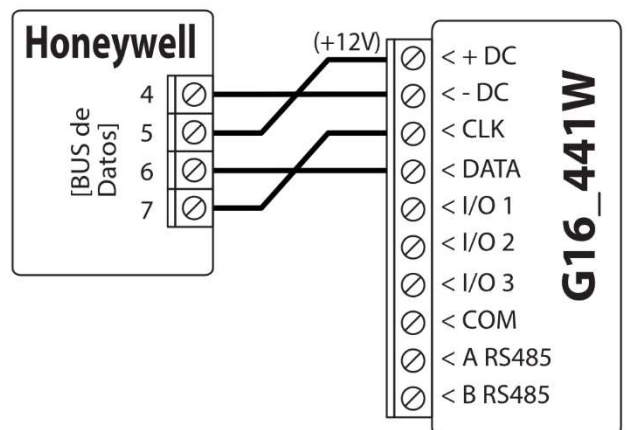
Diagrama de conexión de Honeywell Vista-20, Vista-48 con G16_441W
