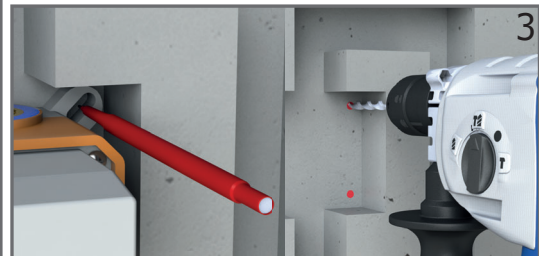
3 MARCAR EN LA PARED LOS HUECOS PARA REALIZAR LOS ORIFICIOS Y TALADRAR MARK THE HOLES ON THE WALL TO MAKE THE HOLES AND DRILL
