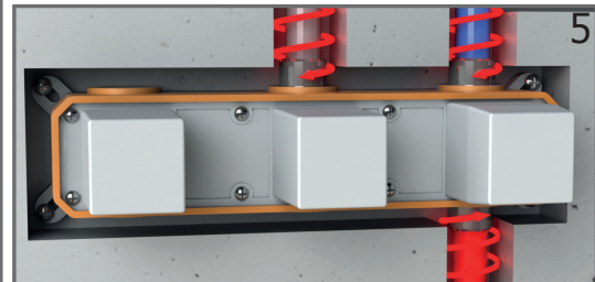
5 INSTALAR LAS TUBERÍAS CON SUS RACORES Y LA CINTA DE TEFLÓN PARA EVITAR FUGAS INSTALL THE PIPES WITH THEIR FITTINGS AND THE TEFLON TAPE TO AVOID LEAKS
