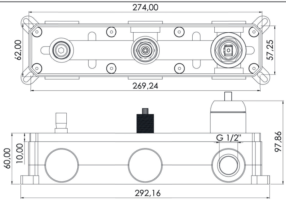
CROKIS CUERPO DE GRIFERIA CROKIS FAUCET BODY
