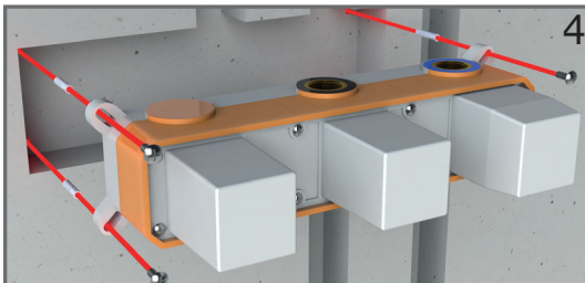
4 COLOCAR LOS TACOS EN LOS ORIFICIOS Y LA CAJA ENCIMA CON TORNILLOS PARA FIJAR LA CAJA A LA PARED PLACE THE PLUGS IN THE HOLES AND THE BOX ON TOP WITH SCREWS TO FIX THE BOX TO THE WALL
