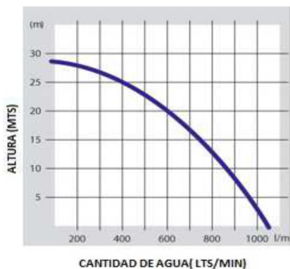
CURVA RENDIMIENTO WB30XH
