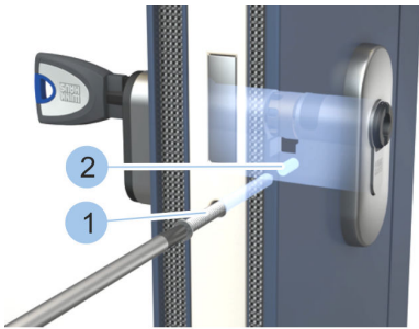
Abb. 45: Zylinder festschrauben
