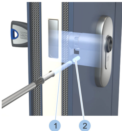
Abb. 37: Stulpschraube einschrauben
