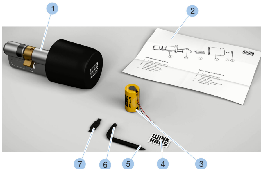
Abb. 139: Batteriewechselset (Typ 04)
