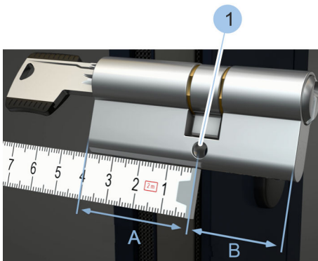
Abb. 27: Alten Zylinder ausmessen
