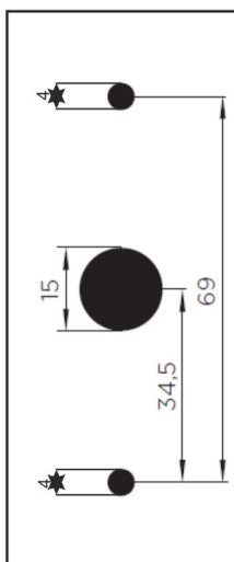
Abb. 166: Bohrbild des Lesers
