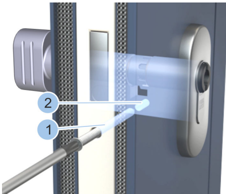
Abb. 41: Zylinder festschrauben
