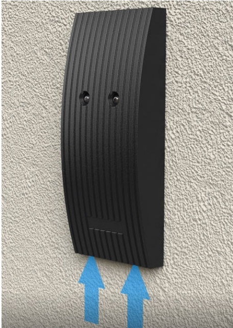
Abb. 126: Lesergehäuse abnehmen
