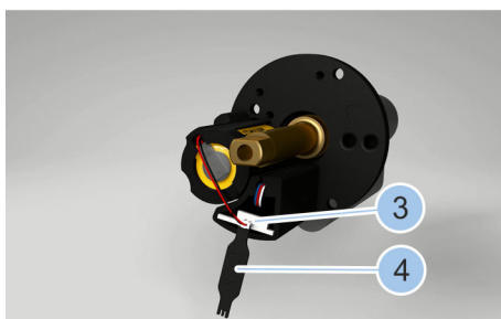
Abb. 144: Schraube und Batteriestecker einsetzen
