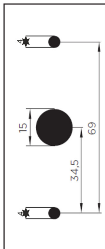
Abb. 167: Bohrbild der Leseinheit
