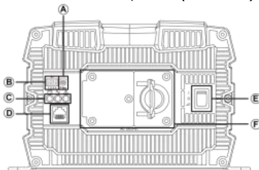
Schéma 9 - SP-3000 / SP-4000 (côté sortie CA)
