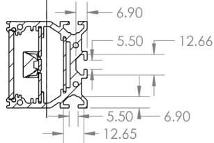
T-SLOT DETAIL SCALE: 1:2
