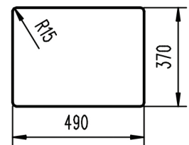
Unterbau 2 bündig
