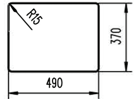
Unterbau 2 bündig
