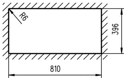
Ausschnitt Unterbau 1:20
