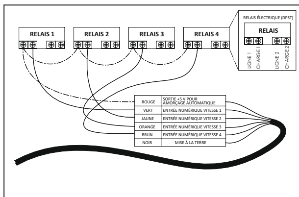
Illustration 4 : Schéma de câblage de l'ensemble de contrôle externe
