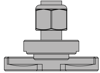
L-TRACK STUD (X2)
