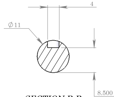
SECTION B-B SCALE 3 : 2
