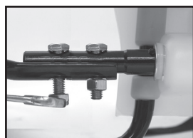
Figure 4 Apriete las tuercas a los pernos
