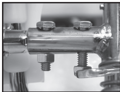
Figure 4 Apriete las tuercas a los pernos
