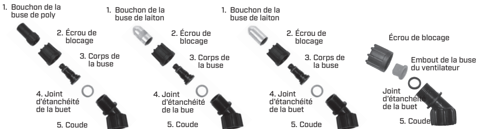
Figure 1 Buse ajustable en polyéthylène
