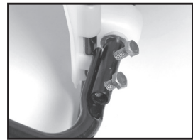
Figure 3 Glisser le boulon à travers les trous
