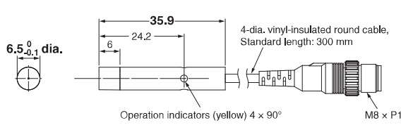
E2E-S05N03-CJ-□□
