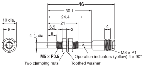
E2E-S05N03-MC-□□
