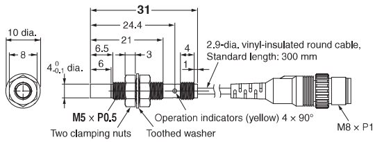
E2E-S05N03-CJ-□□
