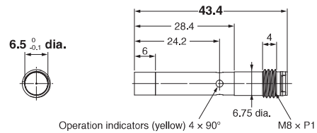
E2E-C06N04-MC-□□
