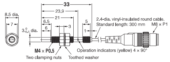
E2E-S04N02-CJ-□□
